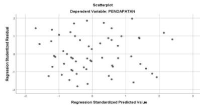
Gambar 2. Grafik Scatterplot
